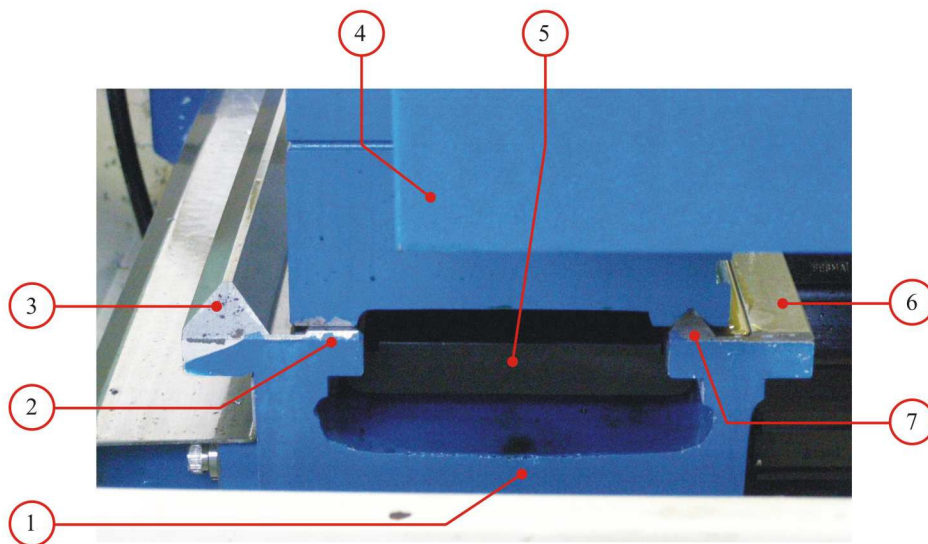
Barramento
