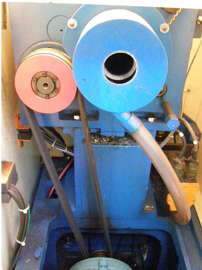
Eixo árvore - Placa - Acionamento e transmissão
