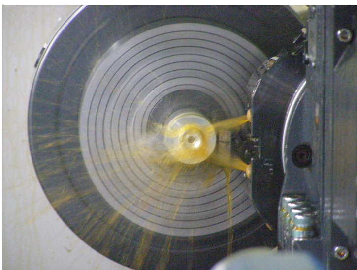
Porta ferramentas
